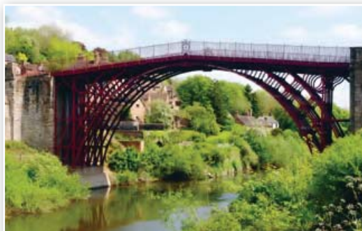
Первый в мире чугунный арочный мост. Великобритания. 1781 г. Памятник Всемирного наследия ЮНЕСКО
